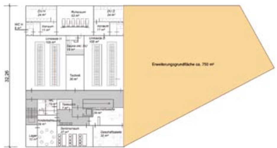
Grundriss 1. Obergeschoss
