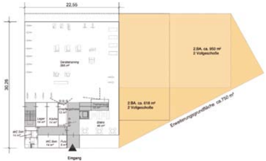
Grundriss Erdgeschoss
