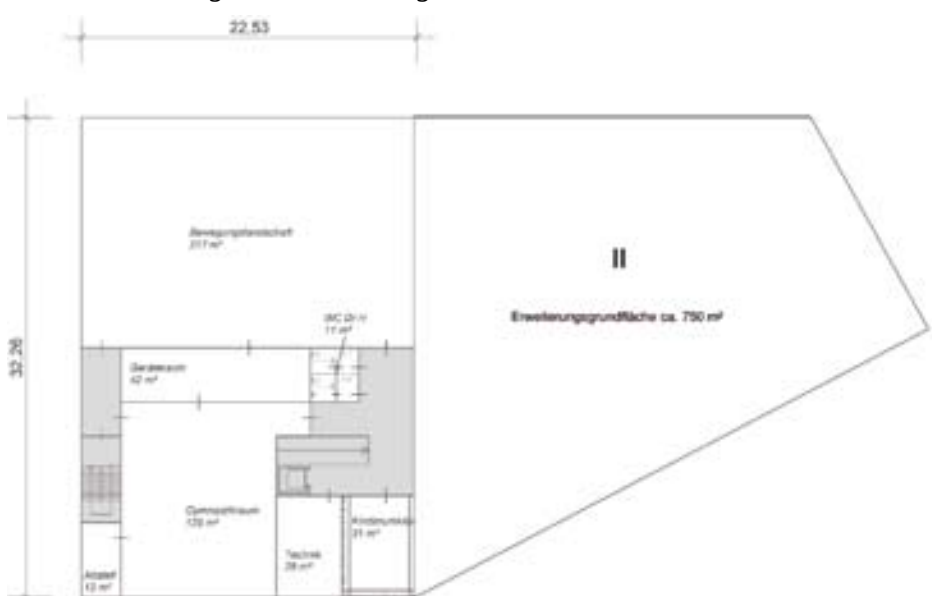
Grundriss 2. Obergeschoss – 3. Obergeschoss = Luftraum
