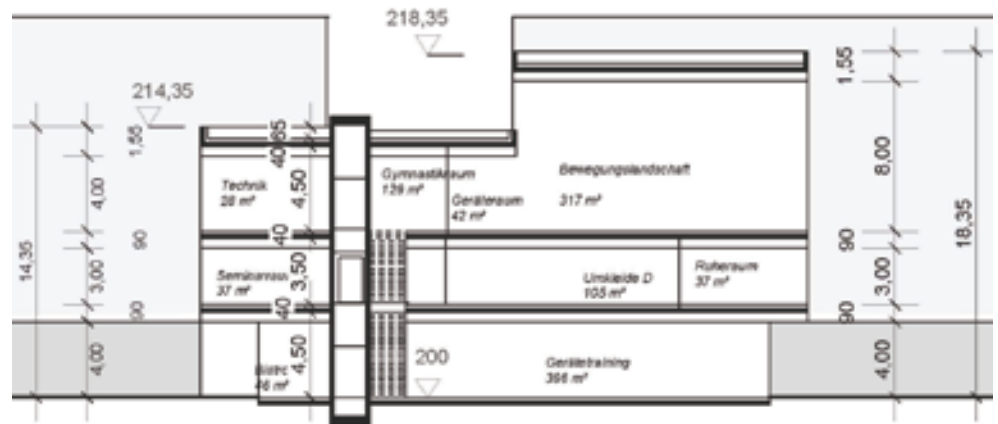
Schnitt – Sicht aus Osten
