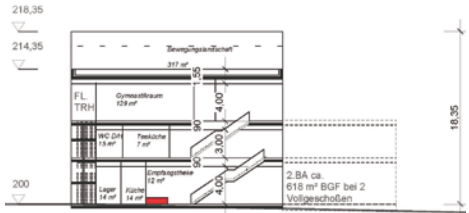
Schnitt – Sicht aus Osten
